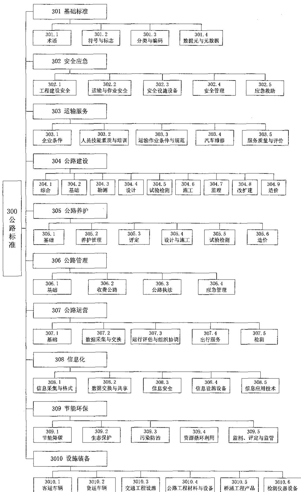
图 6 公路技术标准体系结构图
